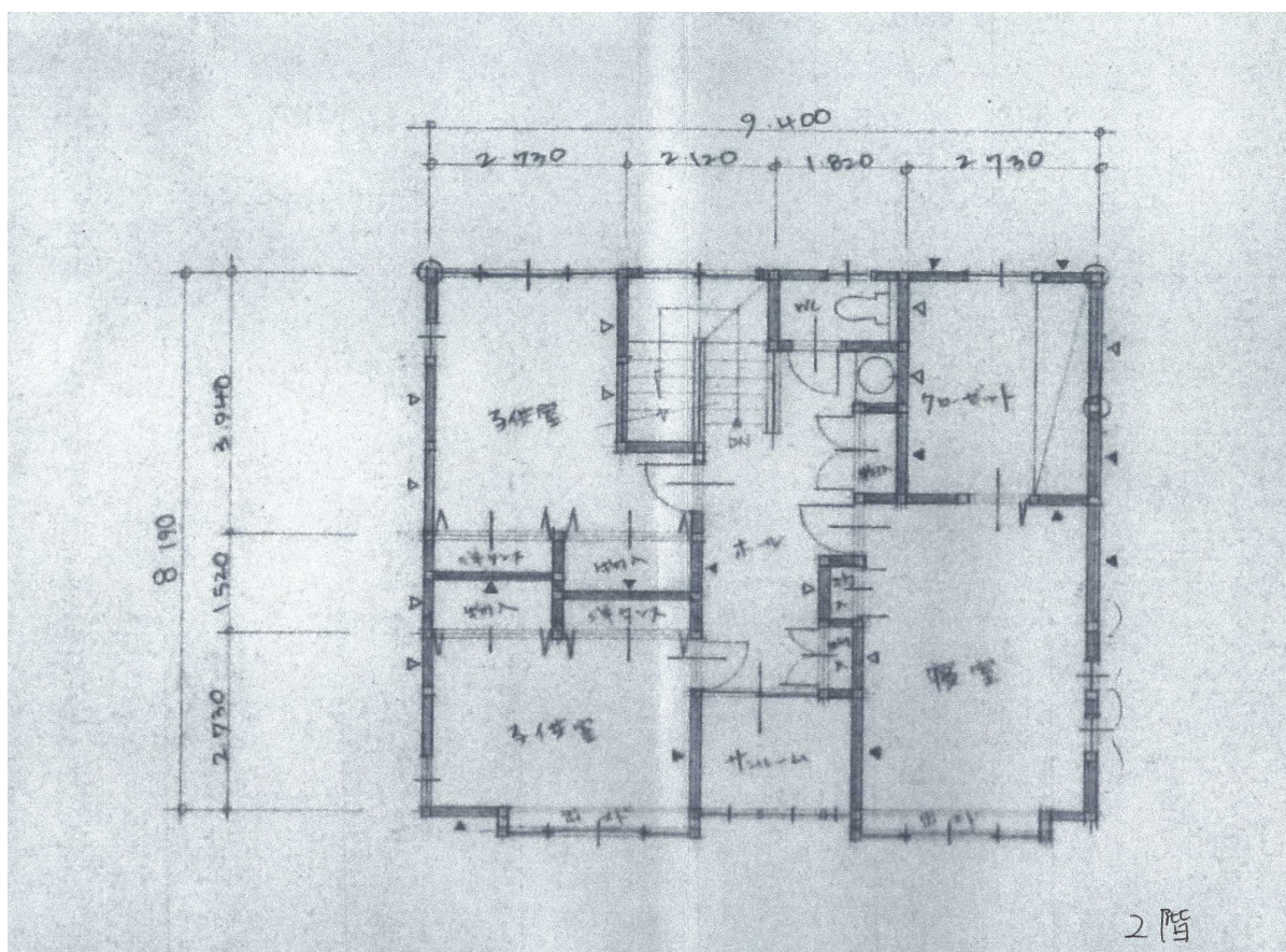
間取り図
